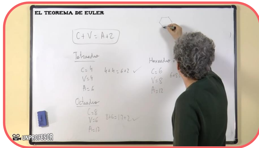
El teorema de Euler
